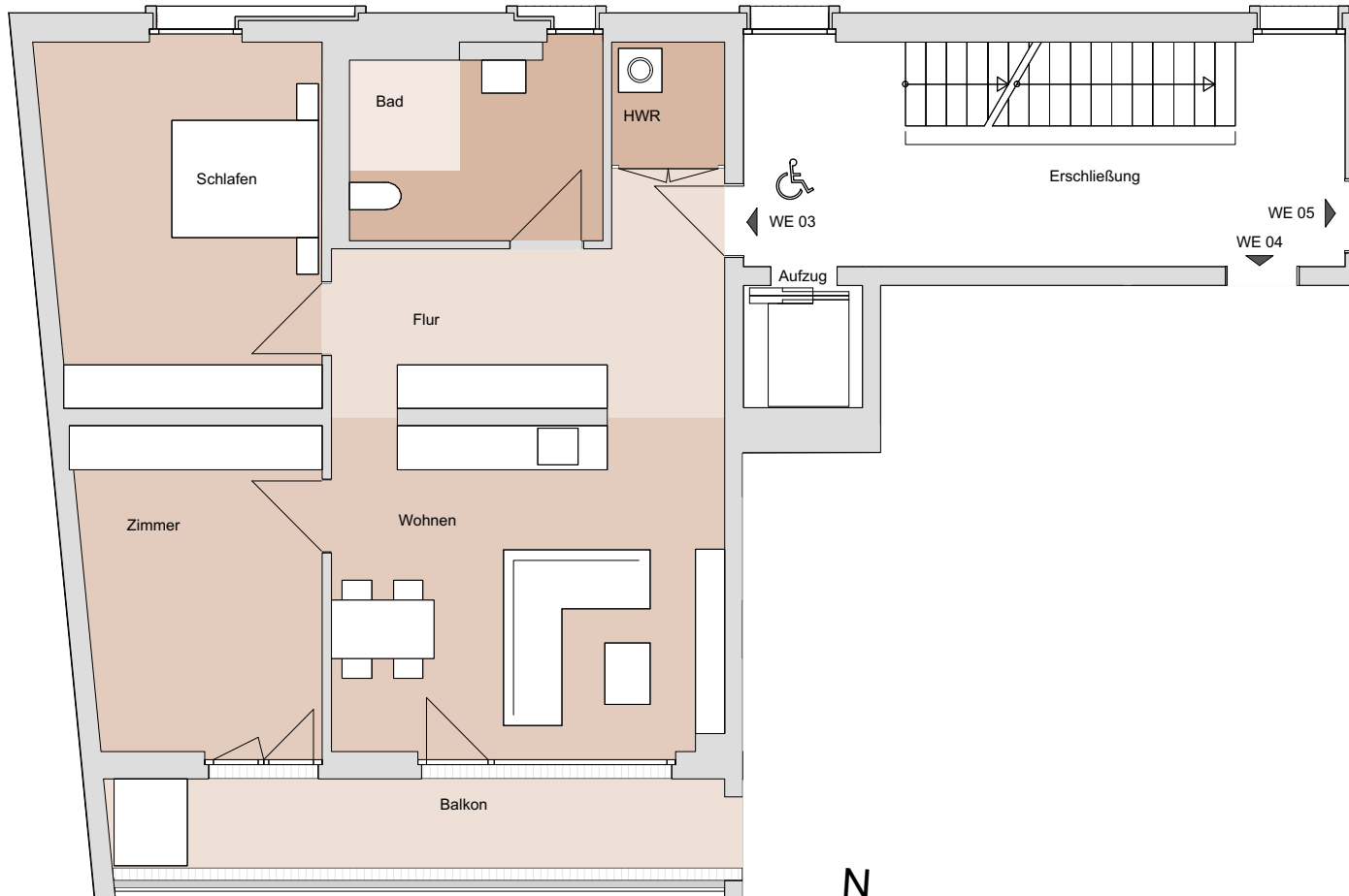
Wohnung 03, 3 Zimmer
